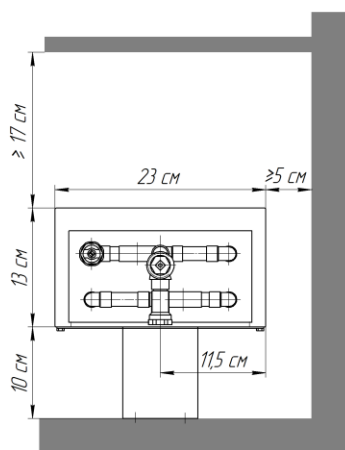
Исполнение "нв" (нерегулируемая высота)
