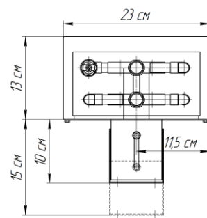
Исполнение "рв" (регулируемая высота)
