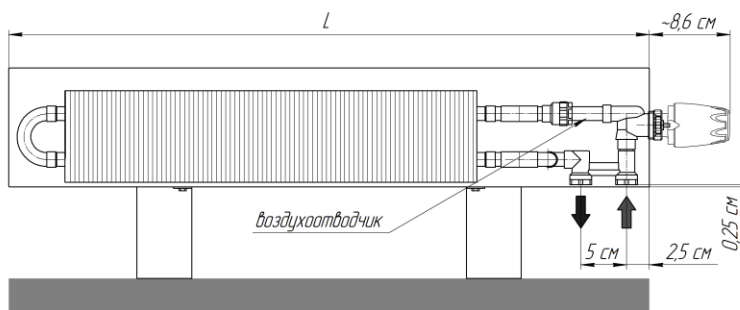
Вид для исполнения "нв" (нерегулируемая высота)
