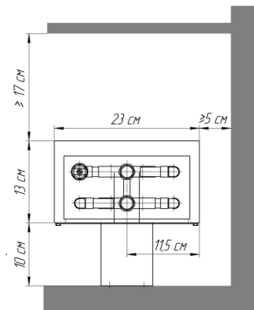
Исполнение "нв" (нерегулируемая высота)
