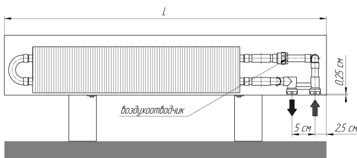
Вид для исполнения "нв" (нерегулируемая высота)
