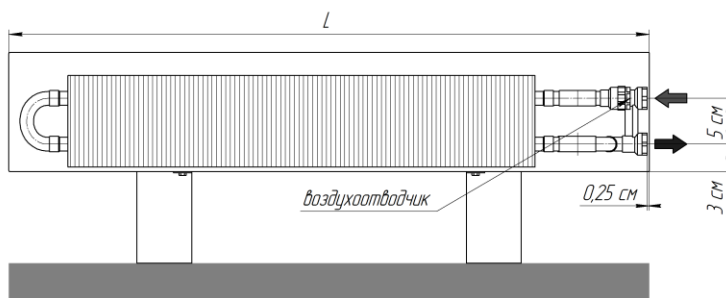
Вид для исполнения "нв" (нерегулируемая высота)
