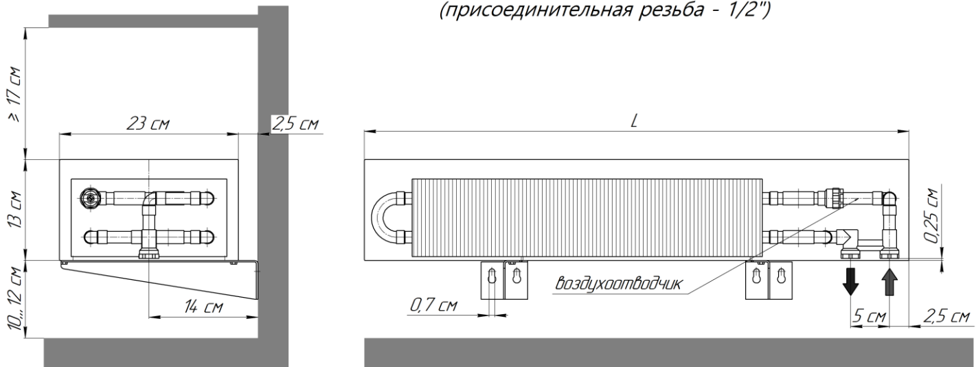
Настенный конвектор "Элегант - мини 230x130-4то Стен прав" с правосторонним нижним подключением (левостороннее - зеркально) (присоединительная резьба - 1/2")
